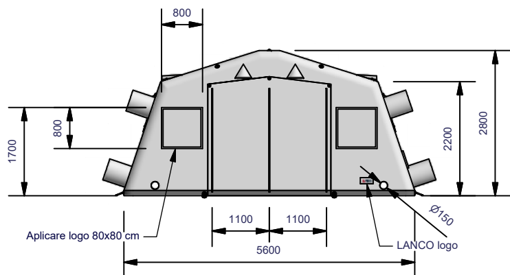
Vedere frontală
